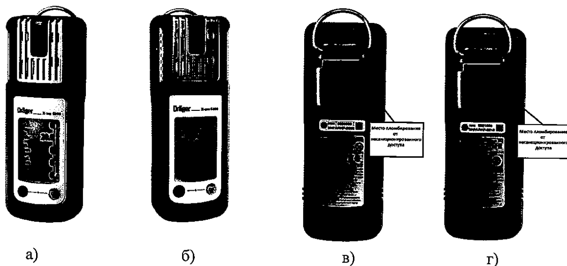
Рисунок 1 – Общий вид газоанализаторов портативных: а) Dräger X-am 5000 тип MQG 0010; б) Dräger X-am 5600 тип MQG 0100; схема пломбирования: в) Dräger X-am 5000 тип MQG 0010; г) Dräger X-am 5600 тип MQG 0100
