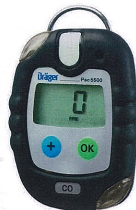
Рисунок 2 – Внешний вид газоанализаторов Dräger Pac модели Pac 5500.
