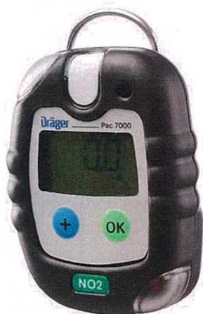
Рисунок 3 – Внешний вид газоанализаторов Dräger Pac модели Pac 7000.
