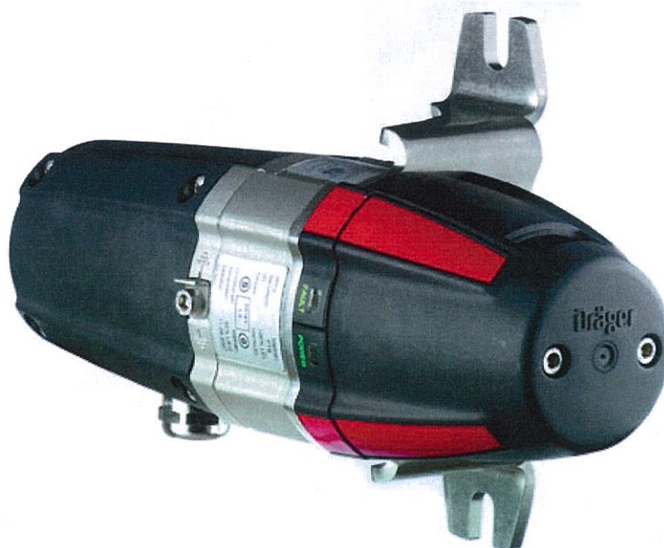
Рисунок 2 – Датчик оптический инфракрасный Dräger модели PIR 7000
